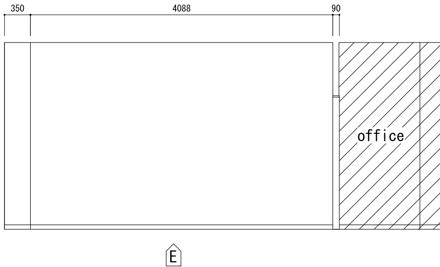
壁面展開図 S1:50
